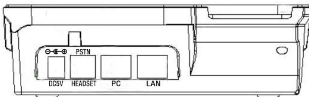
图 2.1 SayHi ES220 系列话机背部连接接口
